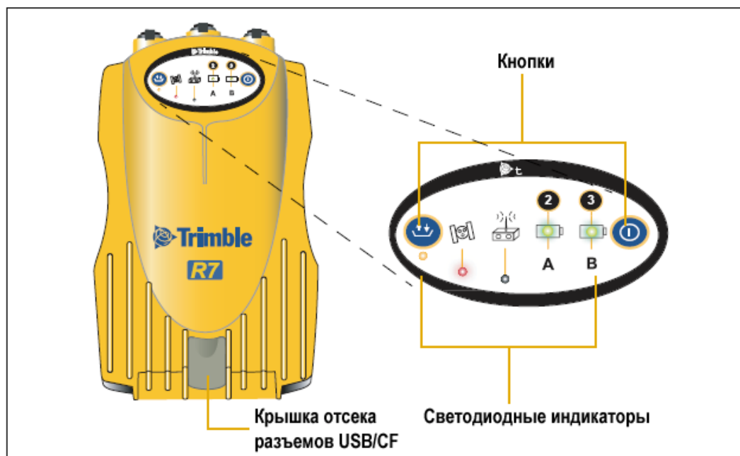
Рис. 3.2 Передняя панель
